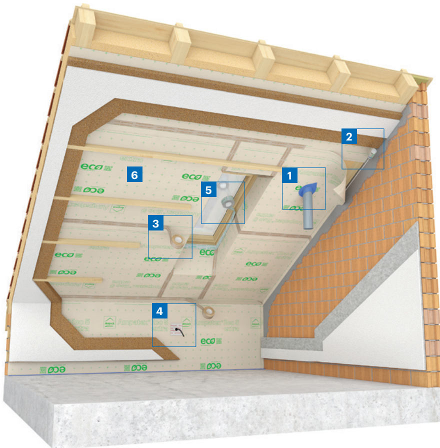
6 Ampatex® Eco 5 extra Bærekraftig damp- brems og lufttett lag
